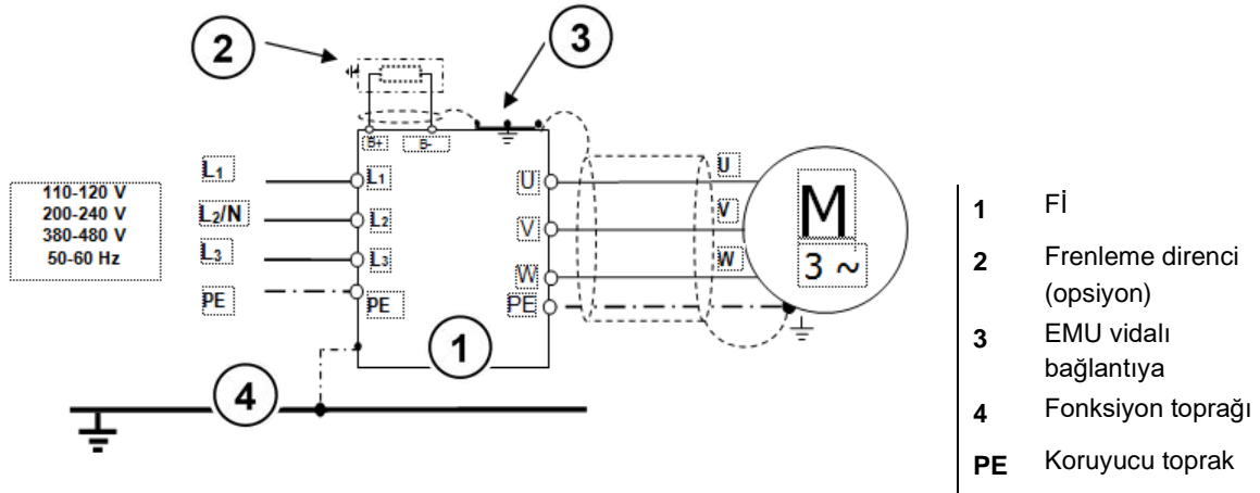
Şekil 33: Kabloleme önerisi
