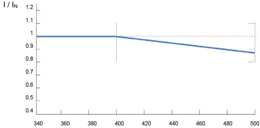
Şekil 35: Şebeke gerilimi sebebiyle azaltılan çıkış akımı
