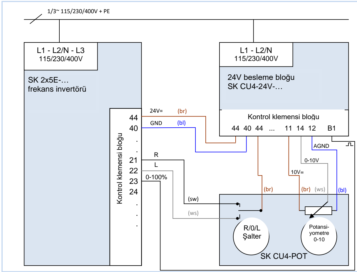
Şekil 26: Bağlantı şeması SK CU4-POT ve parametreleme, örnek SK 2x5E
