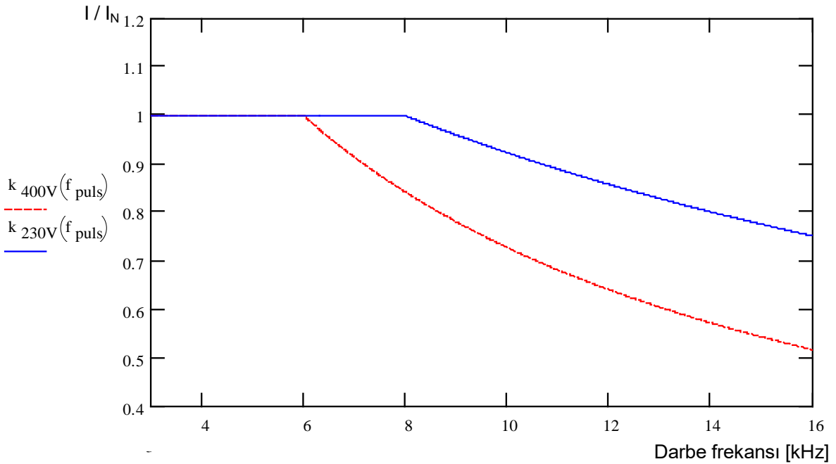
Şekil 34: Darbe frekansı sebebiyle oluşan ısı kayıpları
