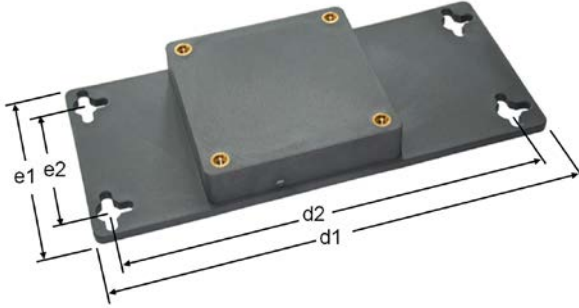
Şekil 8: SK TIE4-WMK-1-K (veya -2-K)
