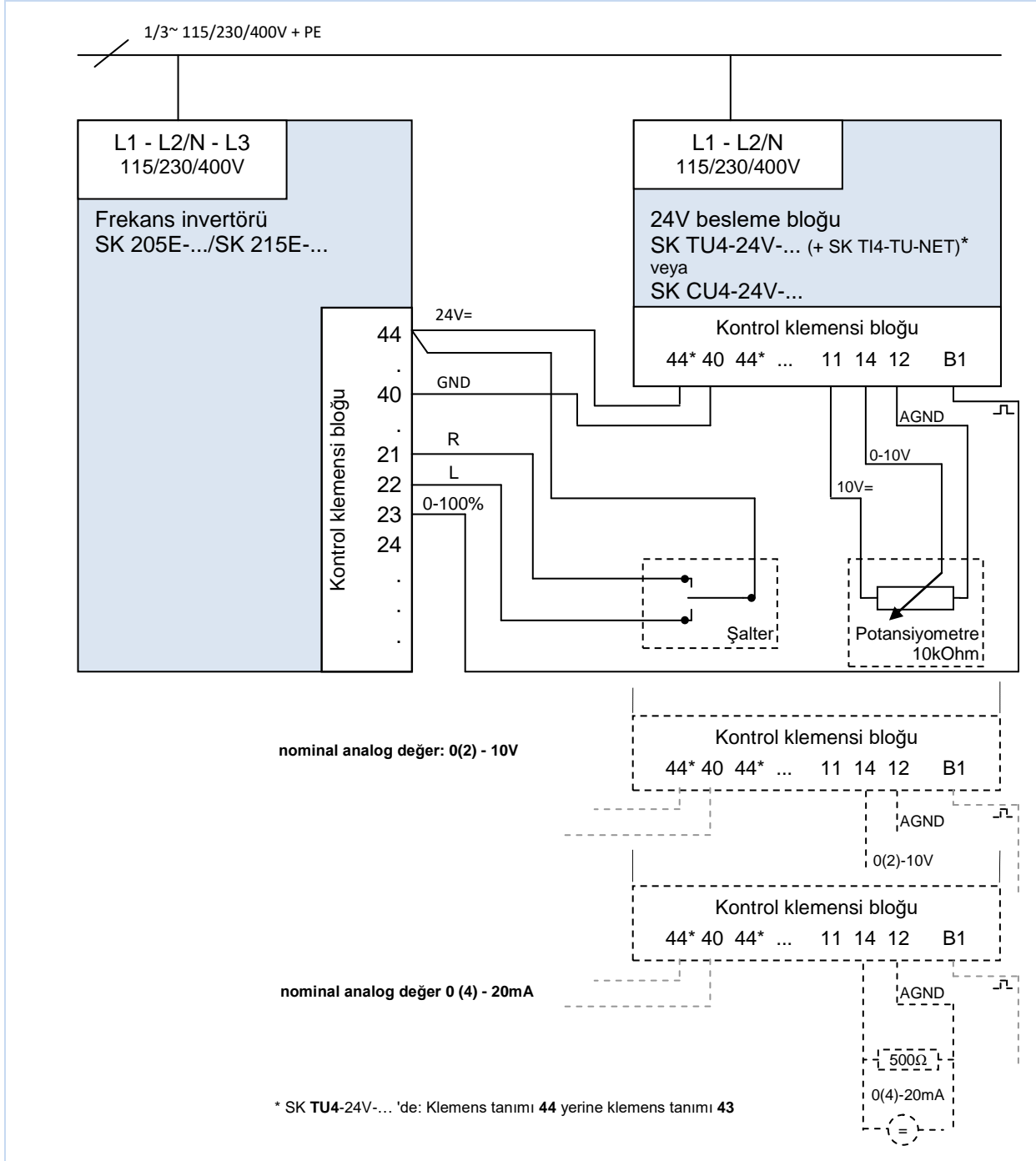
Şekil 17: Besleme bloğu SK xU4-24V-... ile ilgili bağlantı örneği
