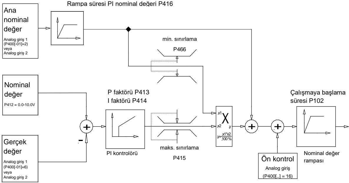
Şekil 32: Proses kontrolörü akış diyagramı
