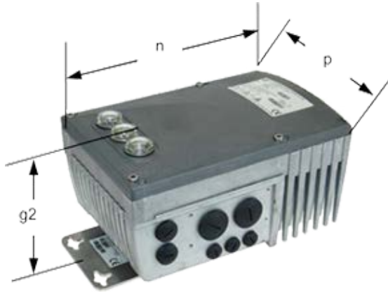
Şekil 10: Duvar montaj kitiyle birlikte SK 2xxE
