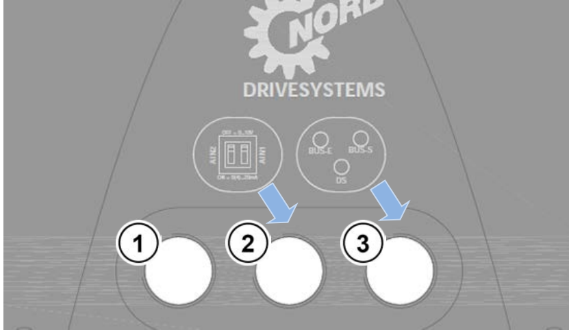
Şekil 29: Arıza teşhis delikleri SK 2x0E (BG 1 ... 3)
