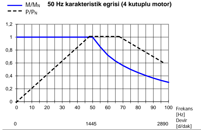
Şekil 38: 50 Hz karakteristik eğrisi
