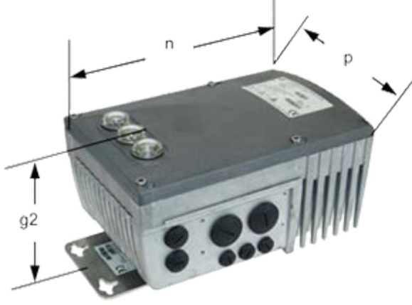
Şekil 7: Duvar montaj kitiyle birlikte SK 2xxE
