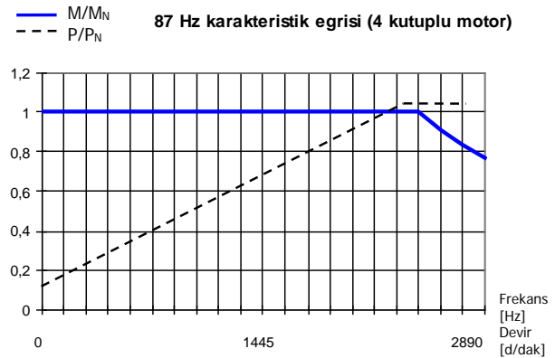
Şekil 39: 87 Hz karakteristik eğri
