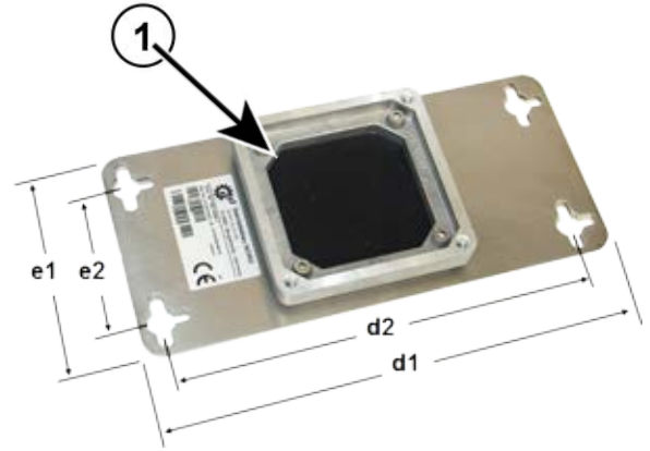
1 Adaptör plakası
