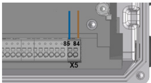
Abbildung 12: Anschlussklemmen AS-i
