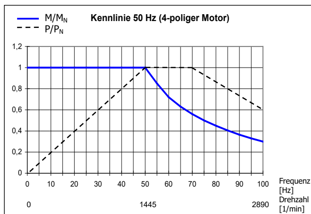
Abbildung 20: Kennlinie 50 Hz
