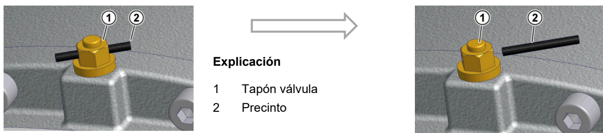
Figura 21: Activación del tapón válvula
