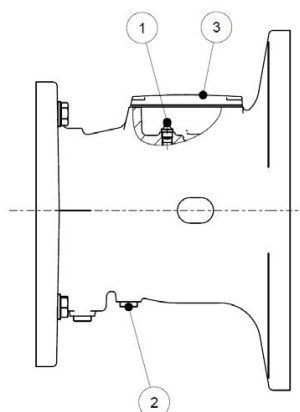
Figura 27: Reengrasar adaptador IEC/NEMA AI y AN opción BRG1
