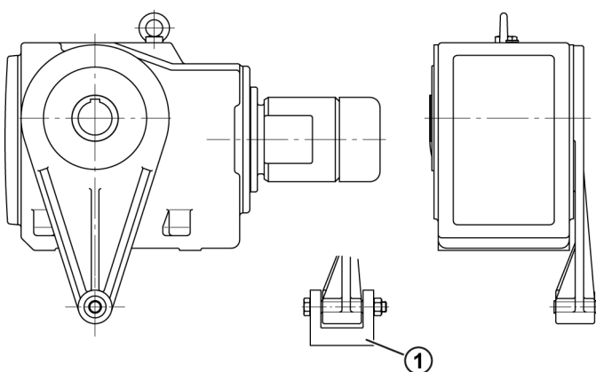
Figura 10: Fijación del brazo de reacción en reductores de engranaje cónico y de sinfín
